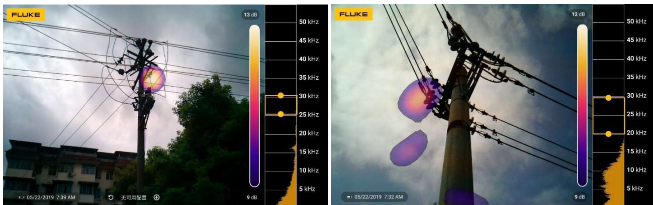
市内10kv线路的绝缘子处的局部放电
